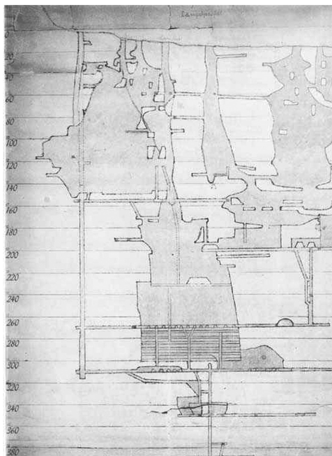
Djupprofil av gruvorna.
