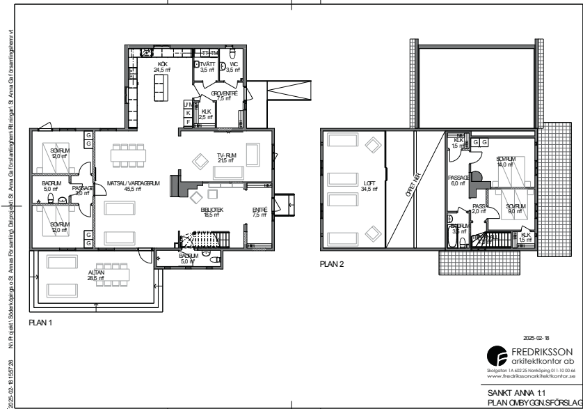
Planer ombyggnadsförslag Sankt Anna gamla församlingshem. Ritning: Fredriksson arkitektkontor AB.
